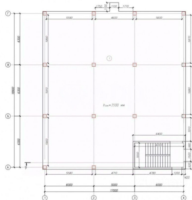
Исполнительная схема ж/б конструкции 2 этажа на отм. +3.950*
