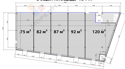
План 1 этажа Общая площадь 464 м 2
