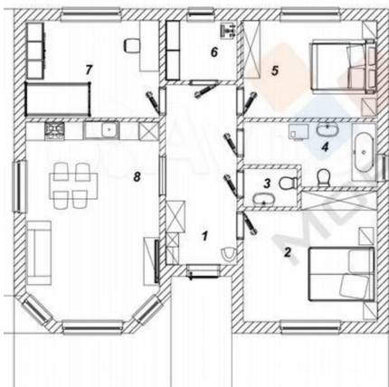
Архитектурный план этажа М1:100
