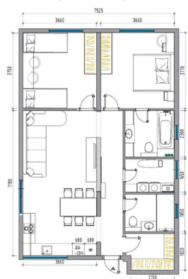
Планировочное решение
