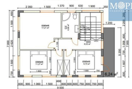
План 2 этажа
