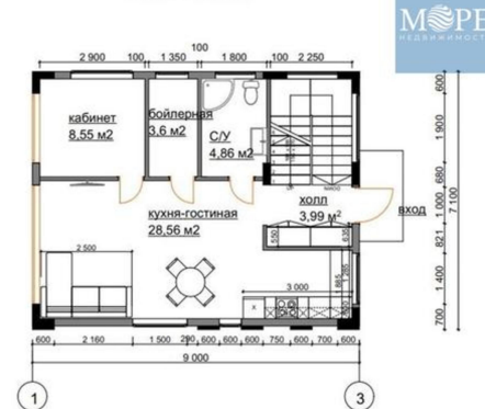
План 1 этажа
